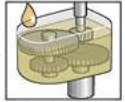
2 kademeli yağ banyolu şanzıman
