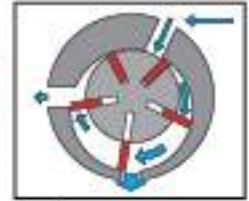
Lamelli motor
