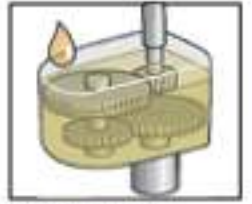
2-kademeli yağ banyosu şanzıman
